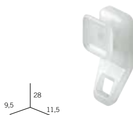
Jednoduchý jezdec "Da-Luz" - přední
