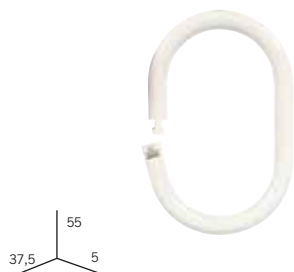
Kroužek koupeľnový, oválný.
